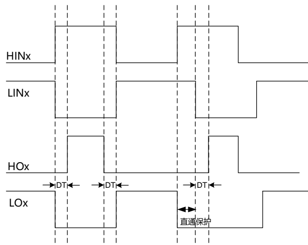
图 5-5 直通保护
