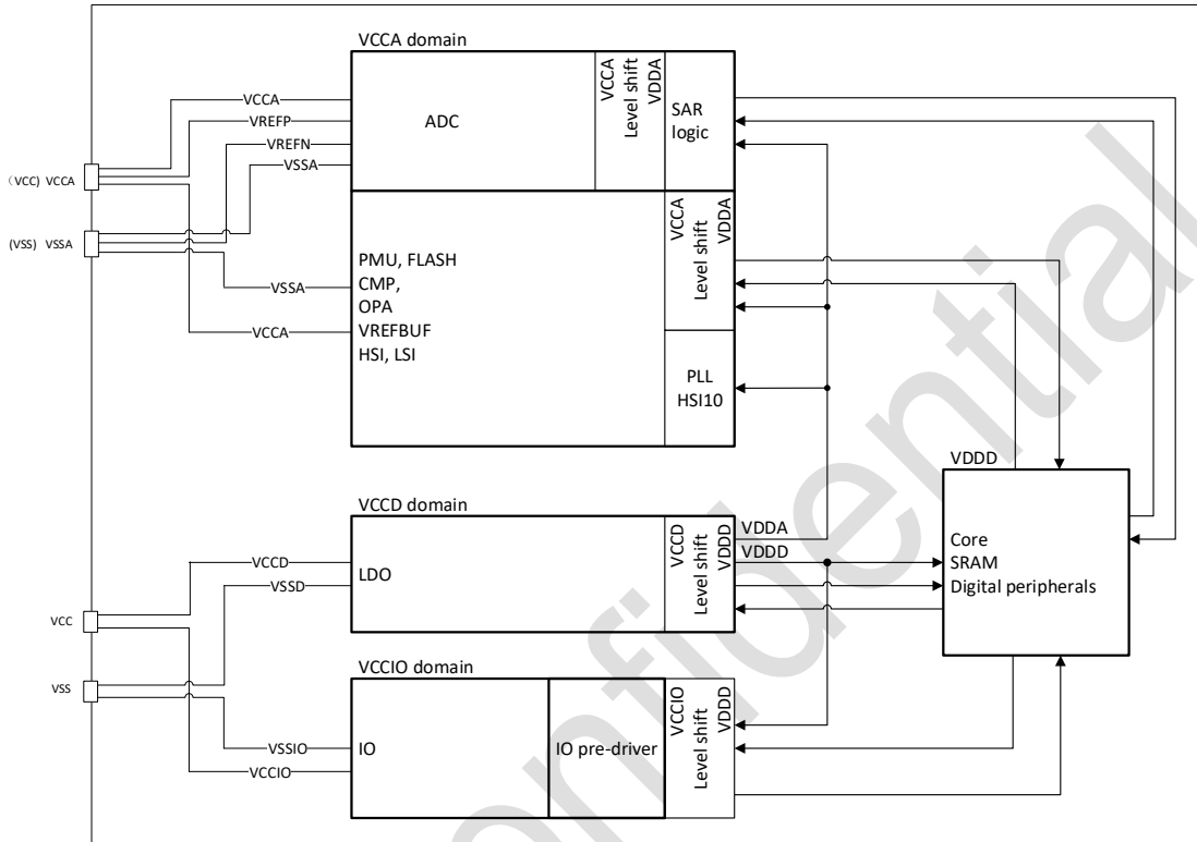
图 2-2 电源框图
