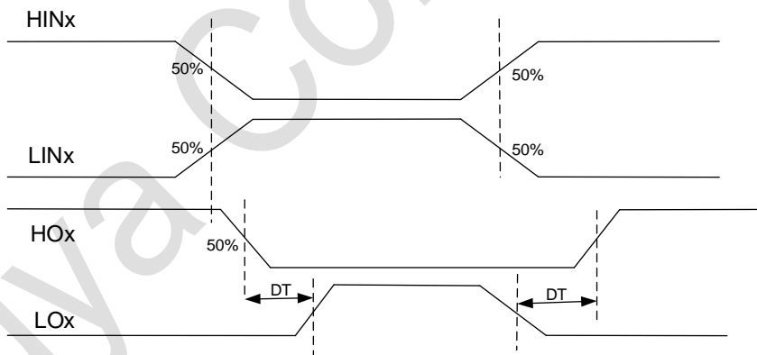
图 5-6 死区功能
