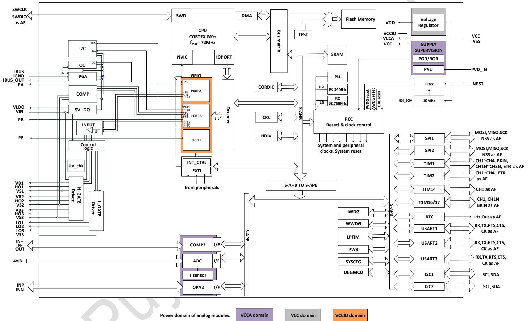
图 1-1 功能模块
