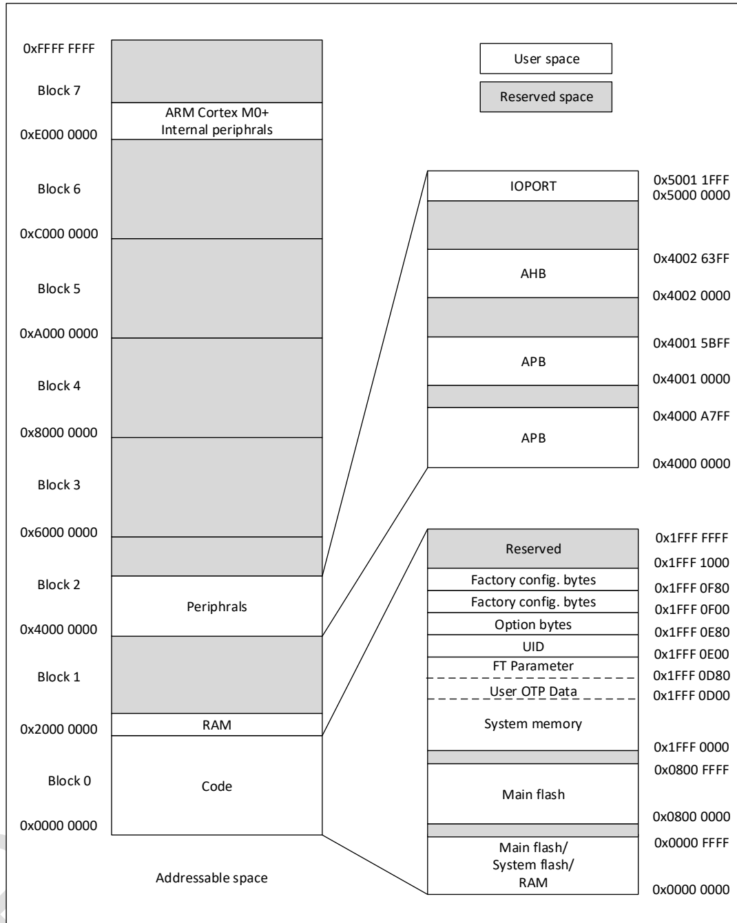
图 4-1 存储器映射
